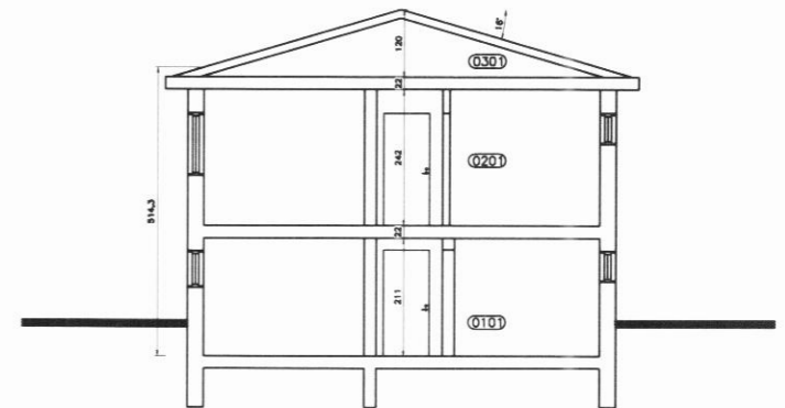
Snid A-A 1:100
