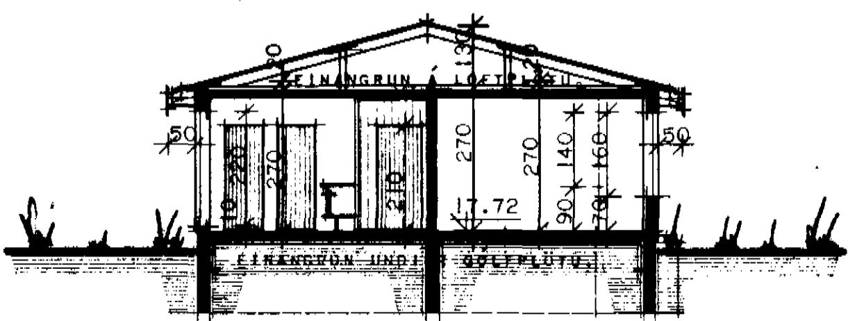
PVERSNÉIDING A-A.
