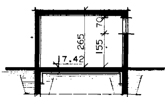
PVERSNÉIDING Í BÍLGEYMSLU
