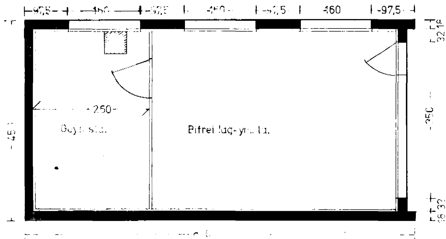
Grundmynd. Mkv. 1:50
