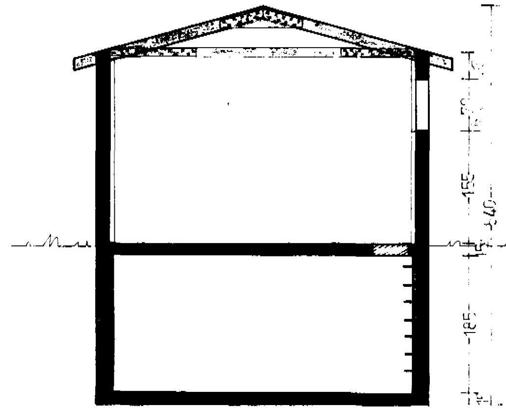
Skurður A-A Mkv. 1:50
