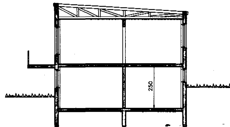
SNID A-A mkv. 1:100
