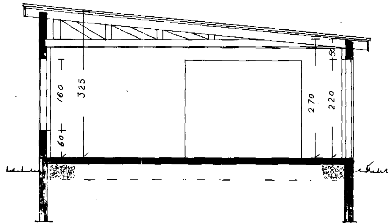
Sneiding A-A M.k.v. 1:50
