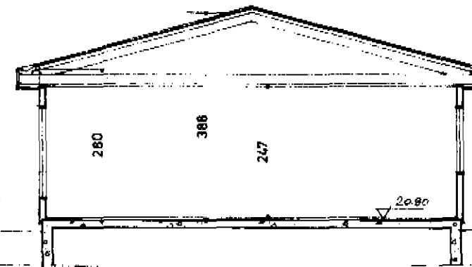
ÞVERSKURÐUR
