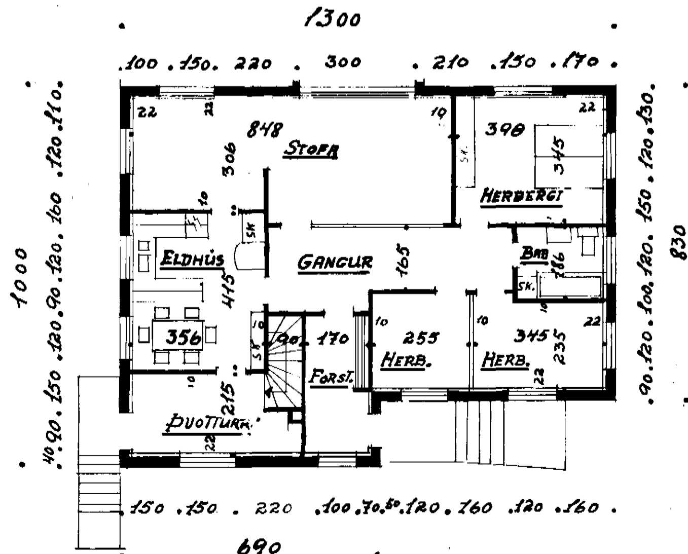
HEÐ
