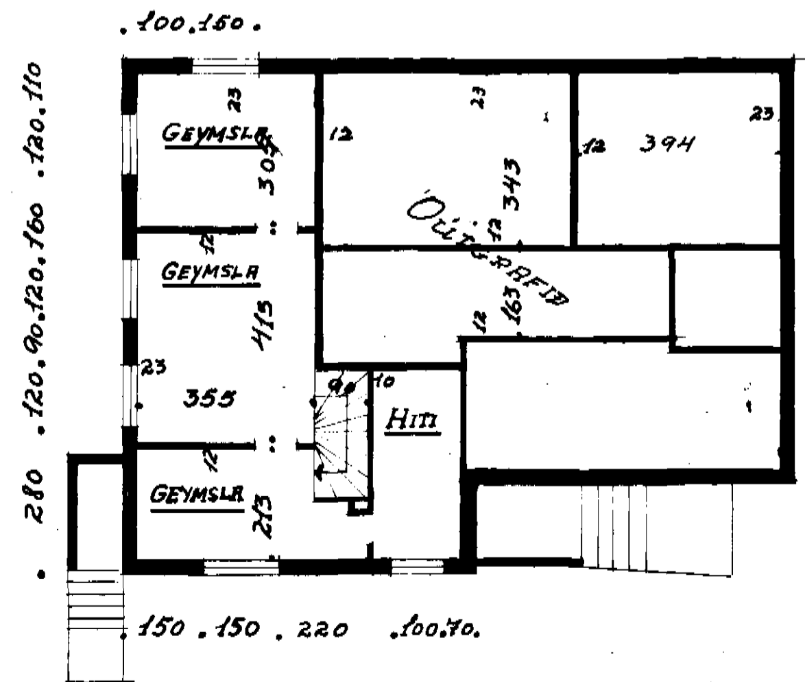
KJALLARI
