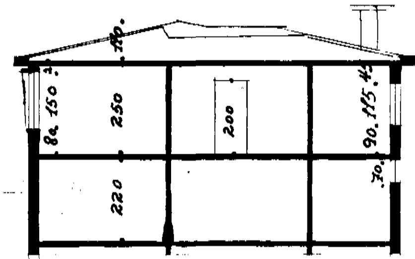
SNEIDING
