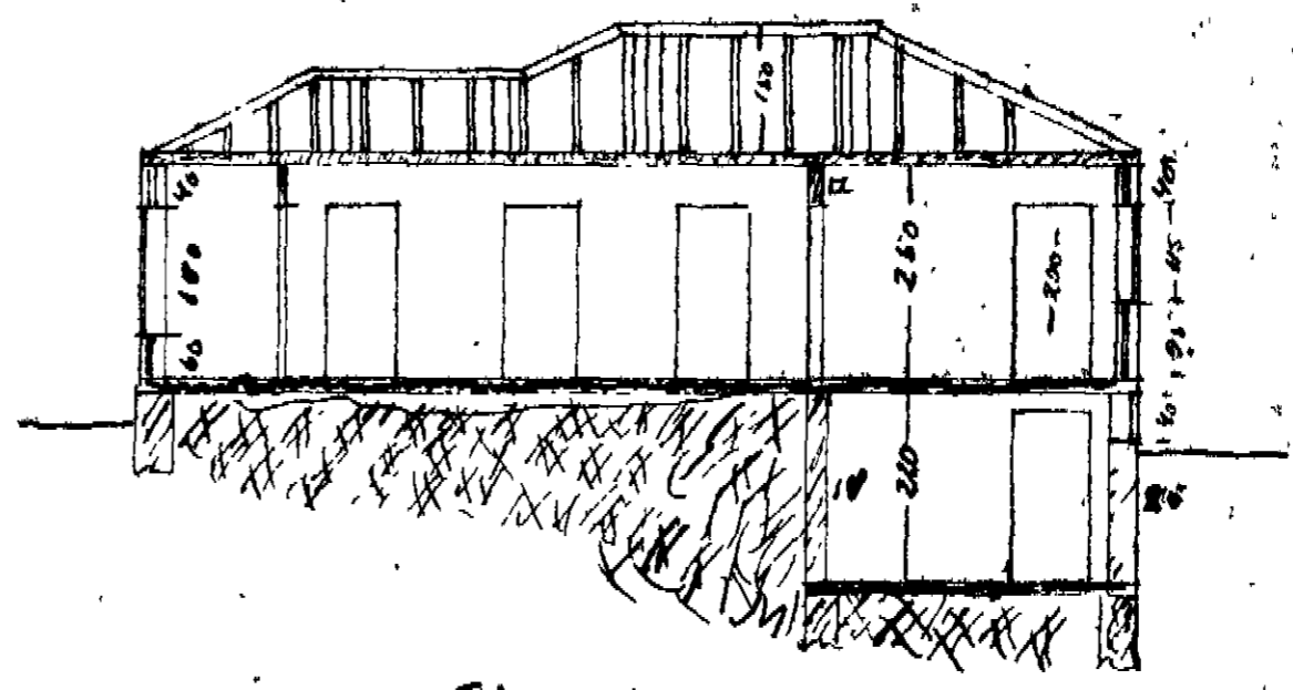
Skurður a-a
