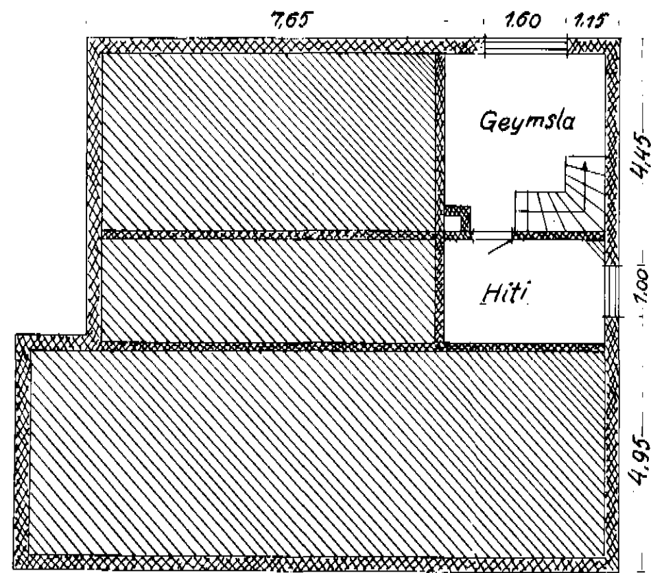
Kjallari
