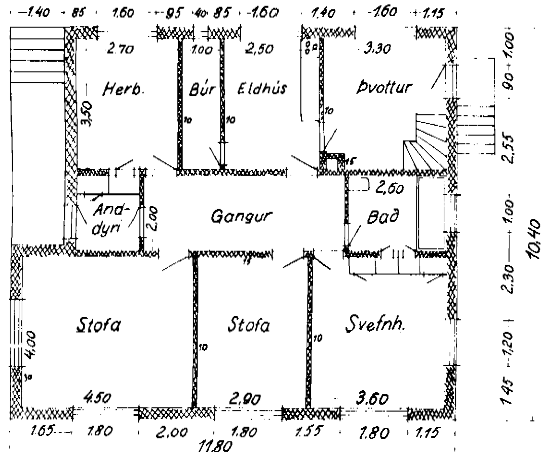
Hæð
