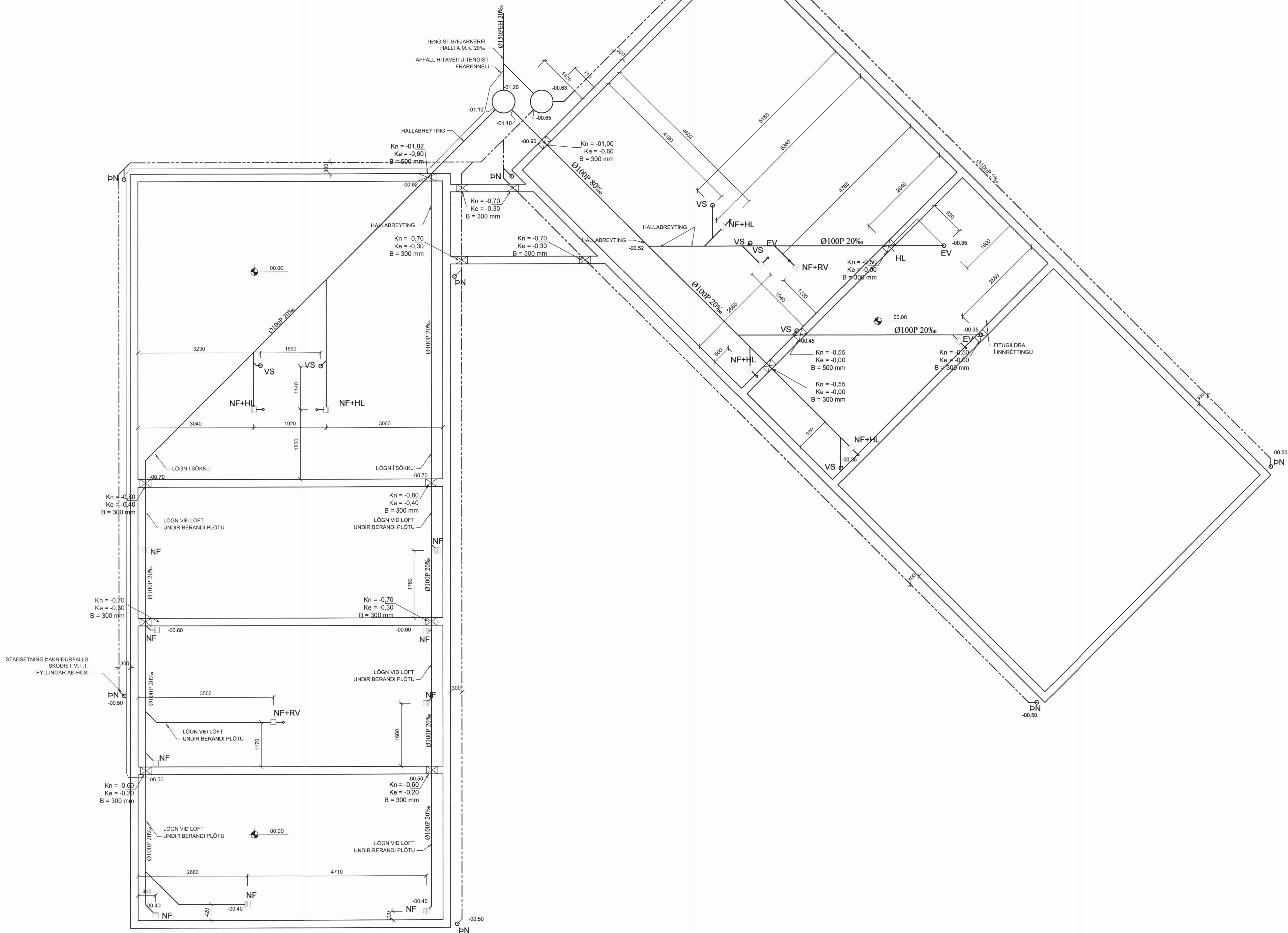
FRÄRENNSLAGNIR Í LAGNAKJALLARA, 1:50 FRÄRENNSLAGNIR Í OG VIÐ SÖKKUL, 1:50
