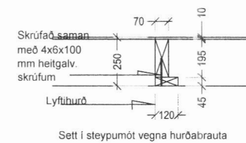
Deili 2, 1:20
