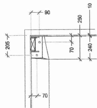
Deili 7, 1:20
