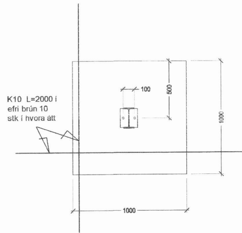
Deili 5, 1:20
