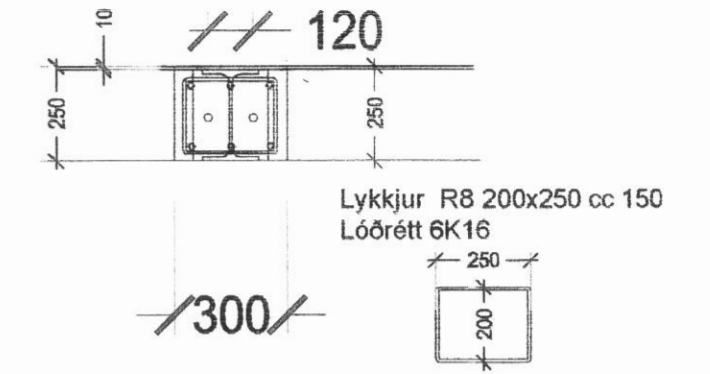
Deili 4, 1:20
