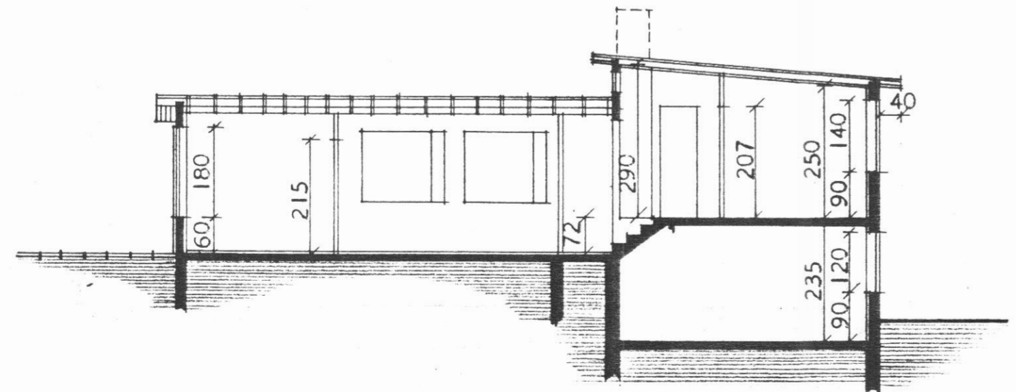
SNEIÐING B - B
