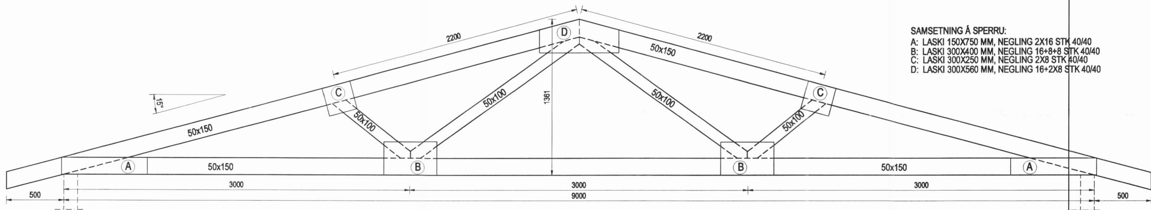
KRASTSPERRA 1 MKV 1:20
